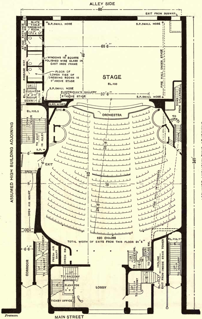
FIG. 21.--MAIN FLOOR PLAN.
